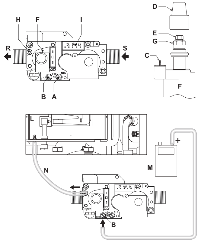
мал. 25 - Газовий клапан
