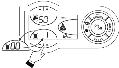
мал. 24 - Режим TEST (потужність опалення = 100%)
