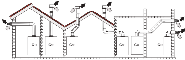
мал. 19 - Приклад підключення за допомогою співісних (коаксіальних) труб (⇨ = Повітря / ⇨ = Відпрацьовані гази)
