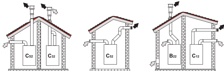
мал. 21 - Приклад підключення за допомогою відокремлених труб (⇨ = Повітря / ⇨ = Відпрацьовані гази)
