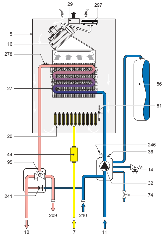
рис. 30 - Схема системы отопления и ГВС
