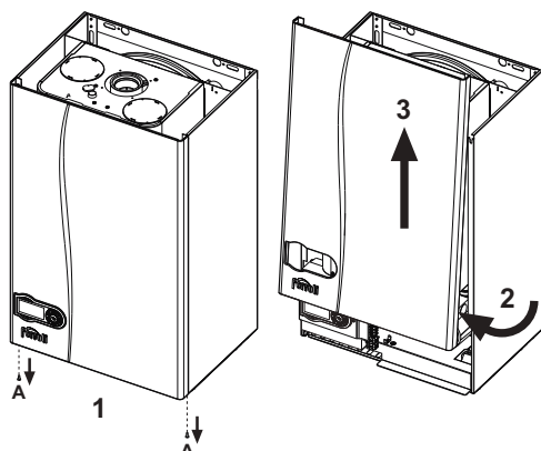
рис. 26 - Снятие кожуха
