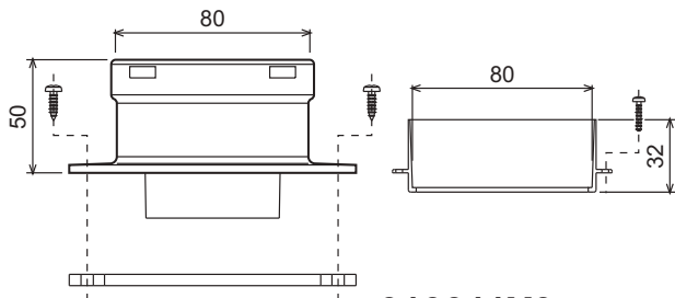
010011X0 мал. 22 - Початковий елемент для відокремлених трубопроводів
