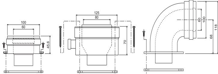
010006X0 010018X0 010007X0 мал. 20 - Початкові елементи для коаксіальних трубопроводів
