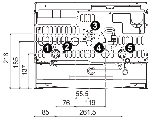
мал. 16 - Гідравлічні штуцери
