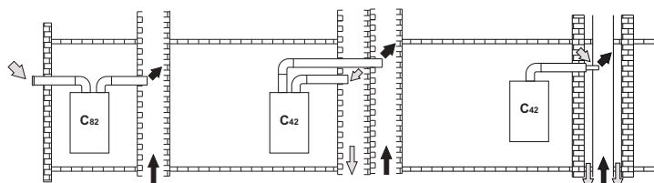
рис. 23 - Примеры подсоединения к дымоходам (⇨ = Воздух / ⇩ = Продукты сгорания)
