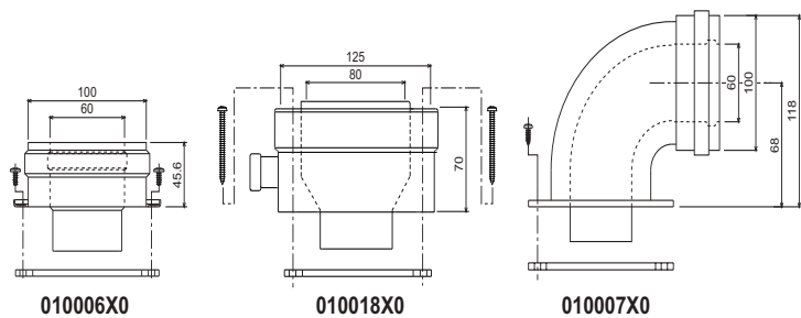
рис. 20 - Исходные элементы для коаксиальных воздухопроводов
